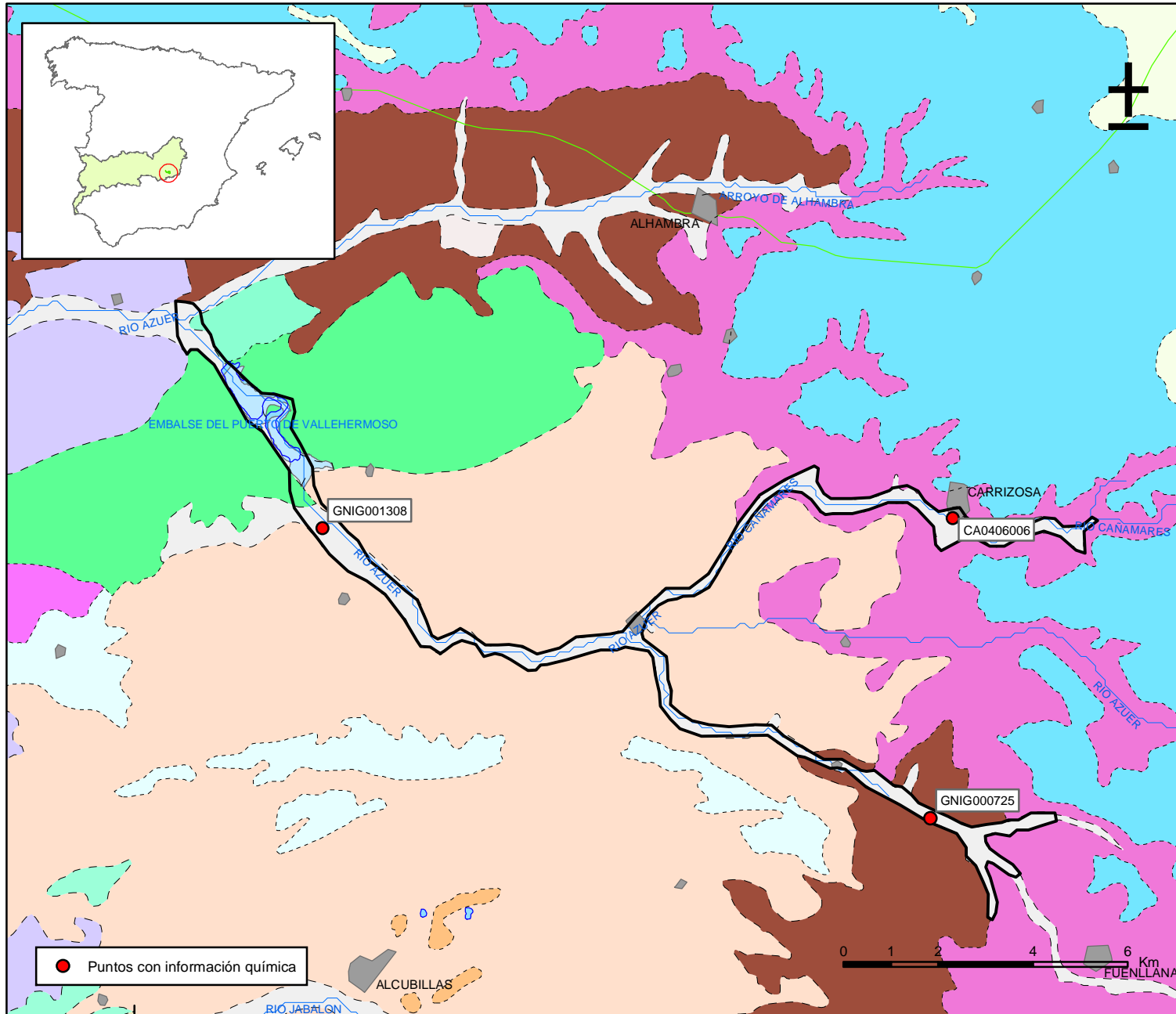
Mapa 10.2. Mapa de calidad química de referencia. Facies hidrogeoquímicas de la masa Aluvial del Azuer (041012)
