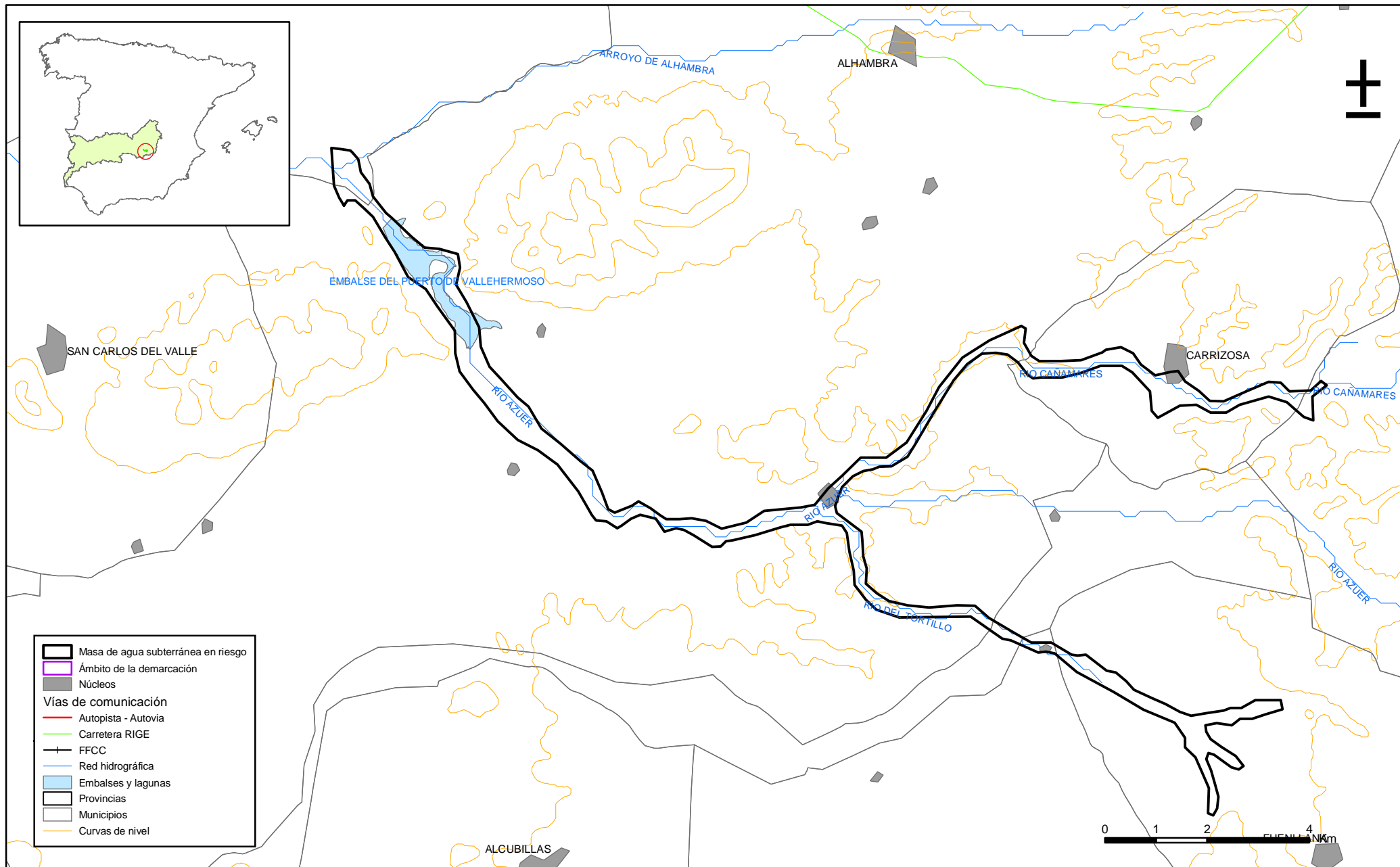
Mapa 1.1. Mapa base cartográfica de la masa Aluvial del Azuer (041012)
