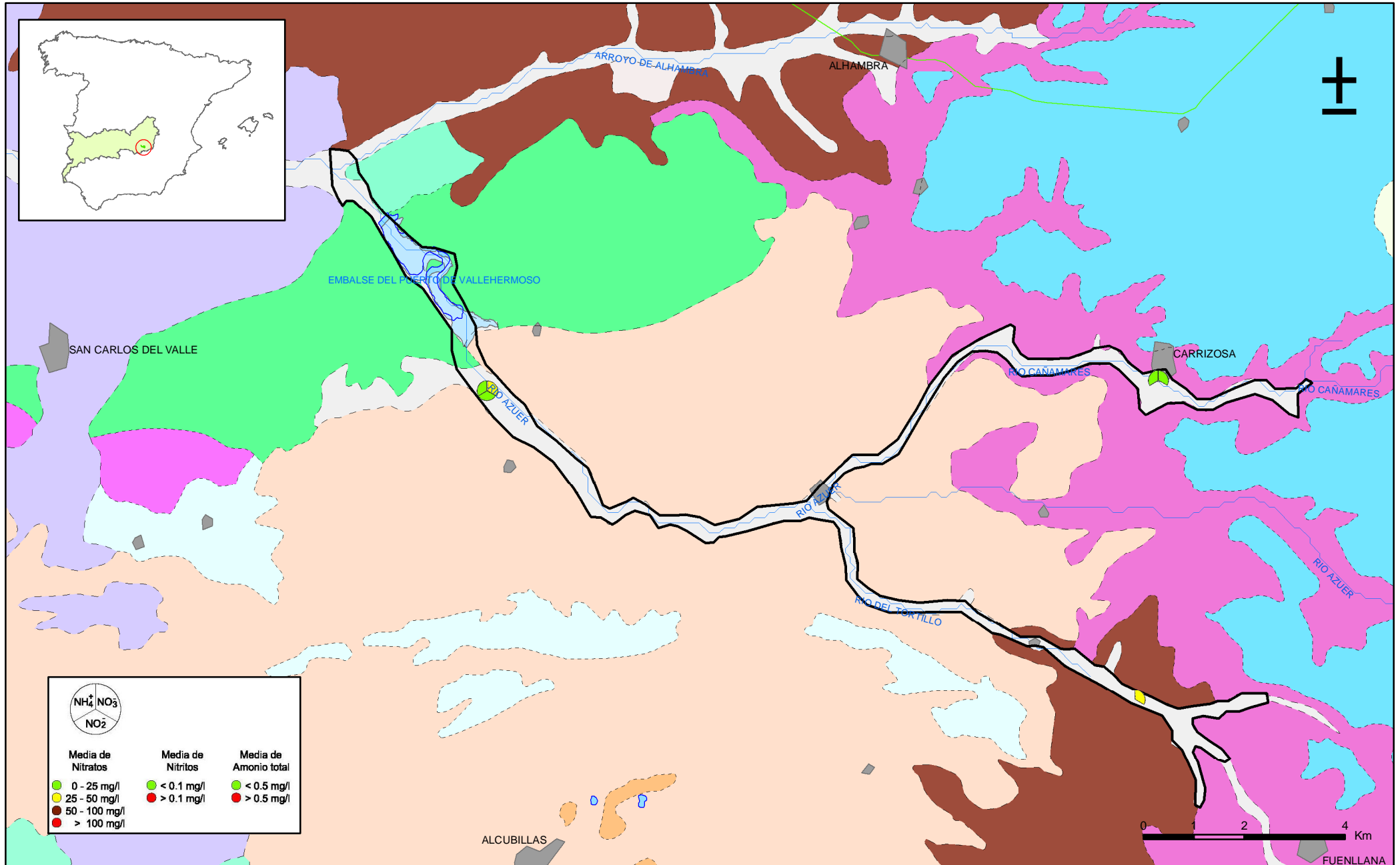
Mapa 10.3.1. Mapa de calidad química de referencia. Compuestos nitrogenados de la masa Aluvial del Azuer (041012)
