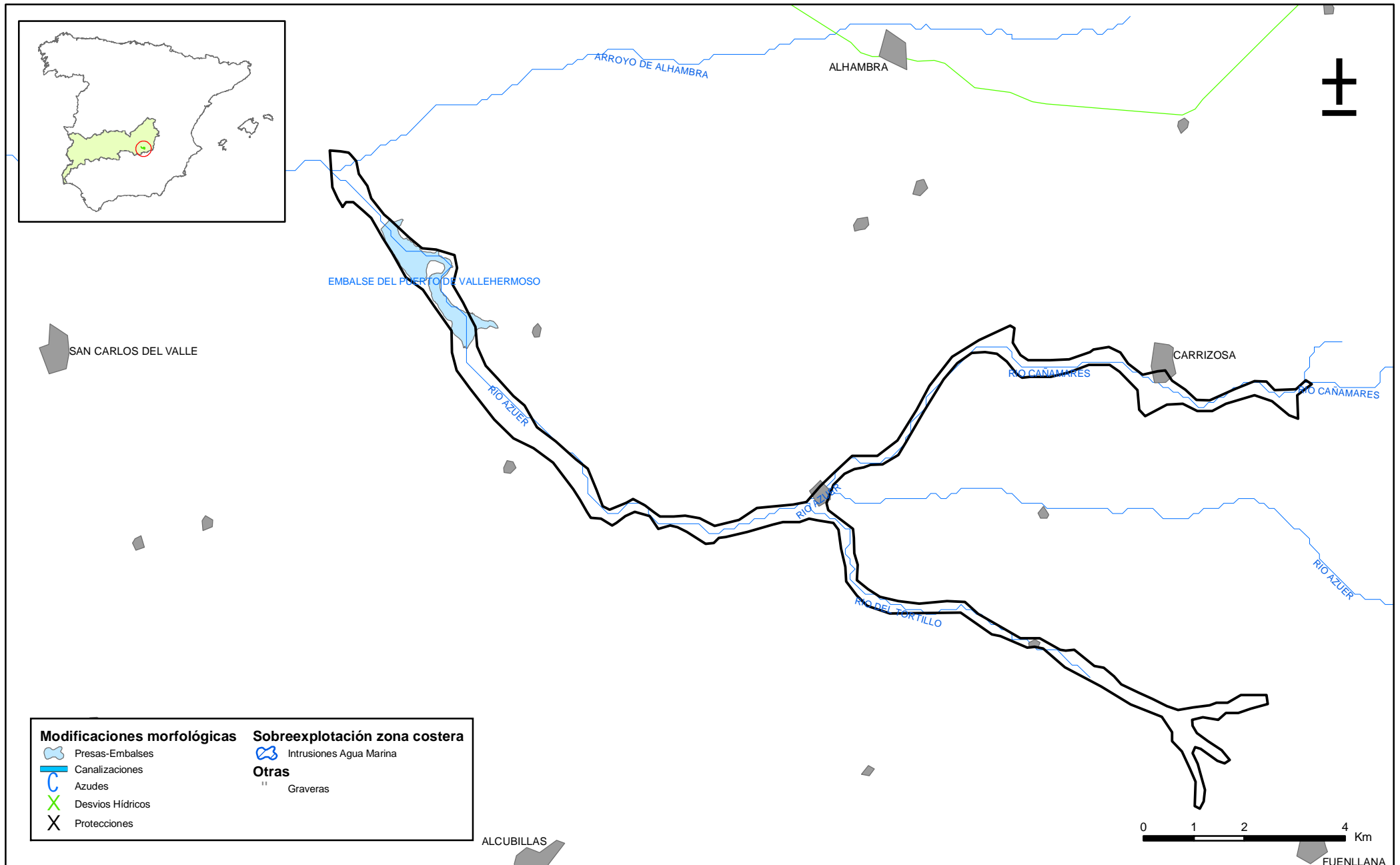
Mapa 15.1. Otras presiones de la masa Aluvial del Azuer (041012)
