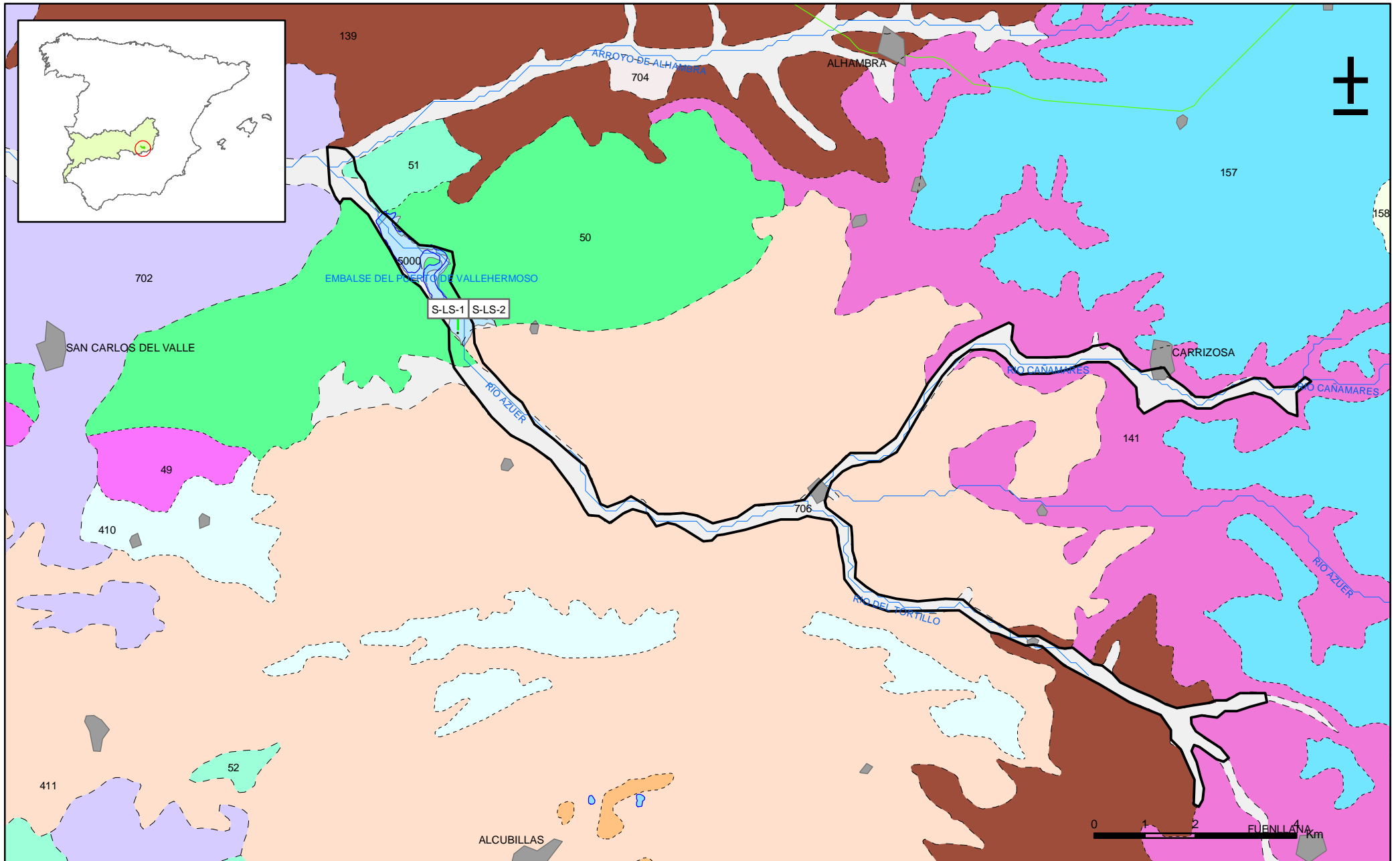
Mapa 2.1. Mapa geológico de la masa Aluvial del Azuer (041012)
