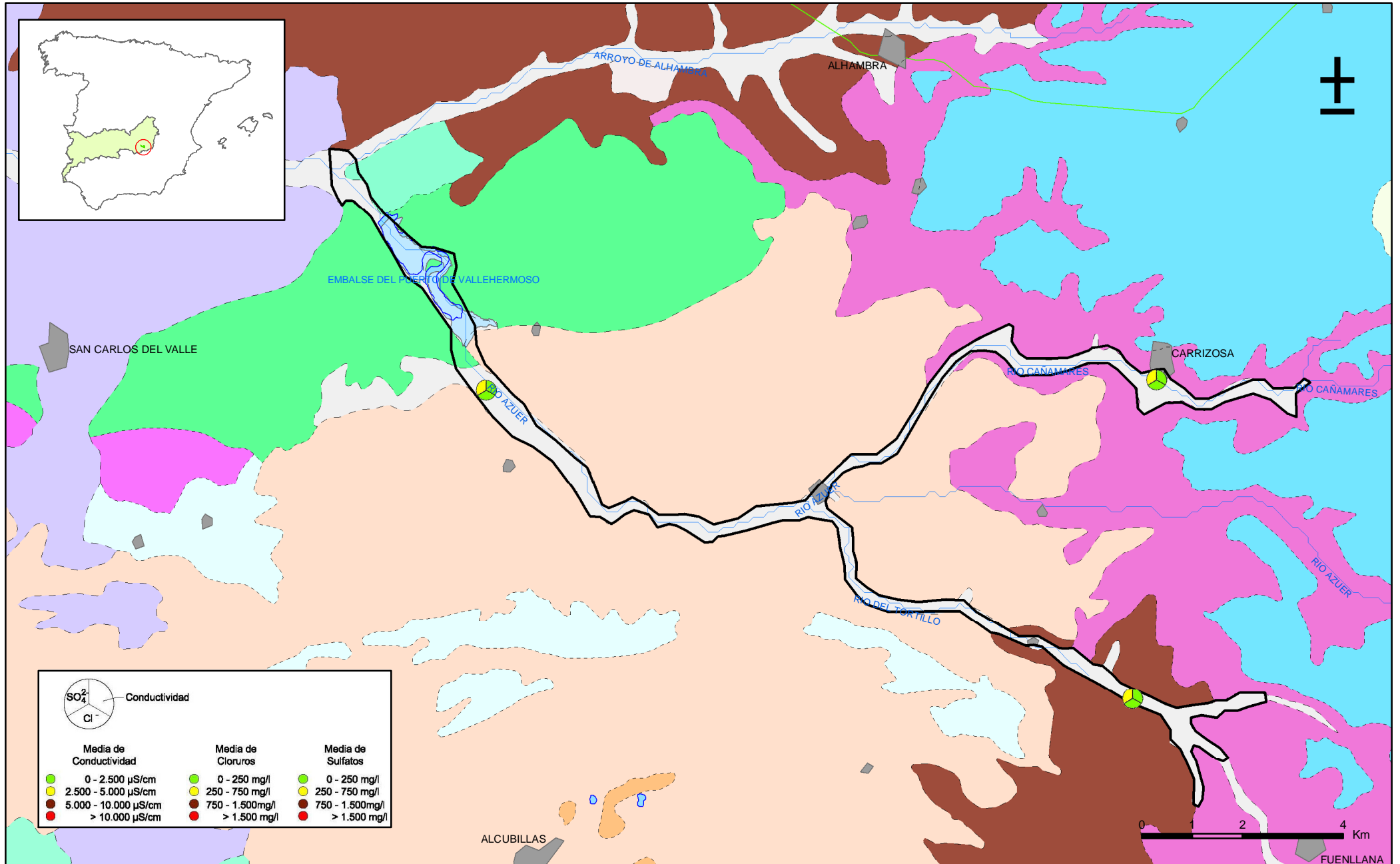
Mapa 10.3.2. Mapa de calidad química de referencia. Conductividad, cloruros y sulfatos de la masa Aluvial del Azuer (041012)
