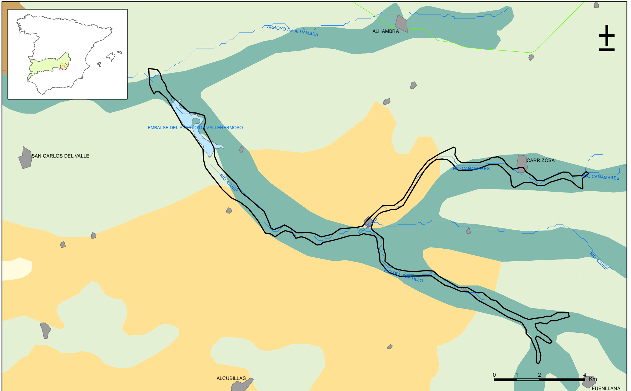
Mapa 4.1. Mapa de suelos de la masa Aluvial del Azuer (041012)
