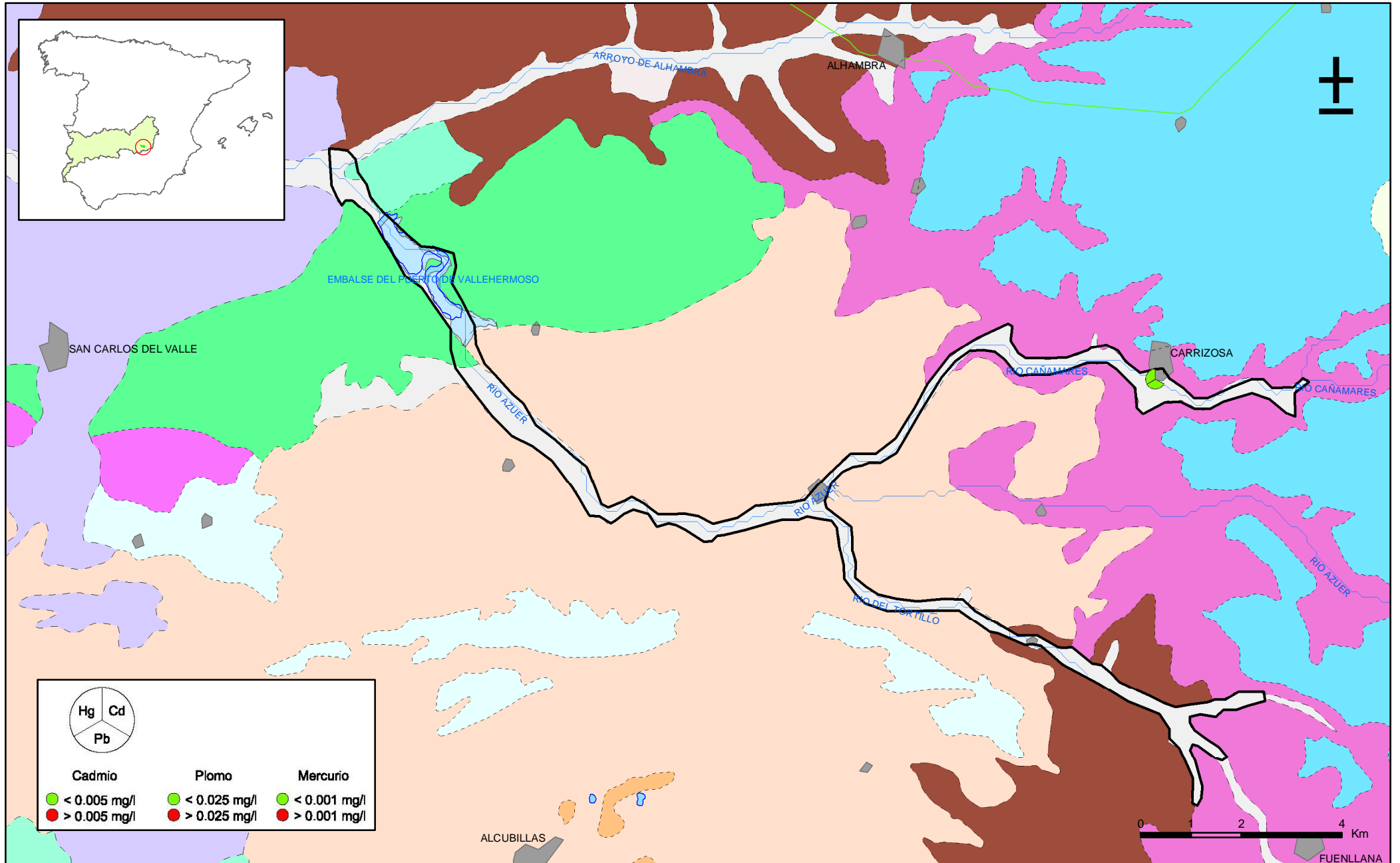
Mapa 10.3.3. Mapa de calidad química de referencia. Metales de la masa Aluvial del Azuer (041012)
