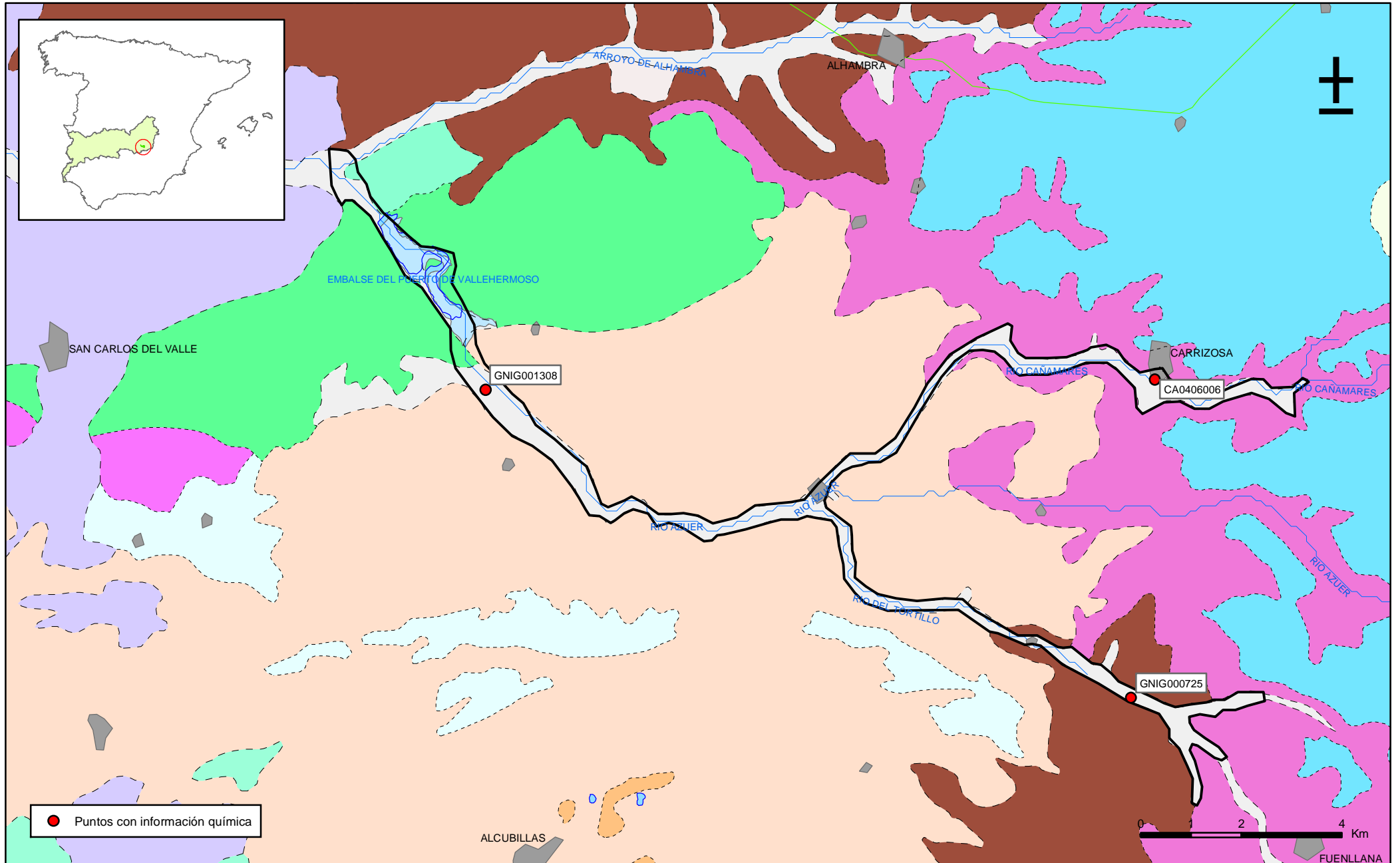
Mapa 10.1. Mapa de situación de puntos utilizados en la determinación de niveles de referencia de la masa Aluvial del Azuer (041012)
