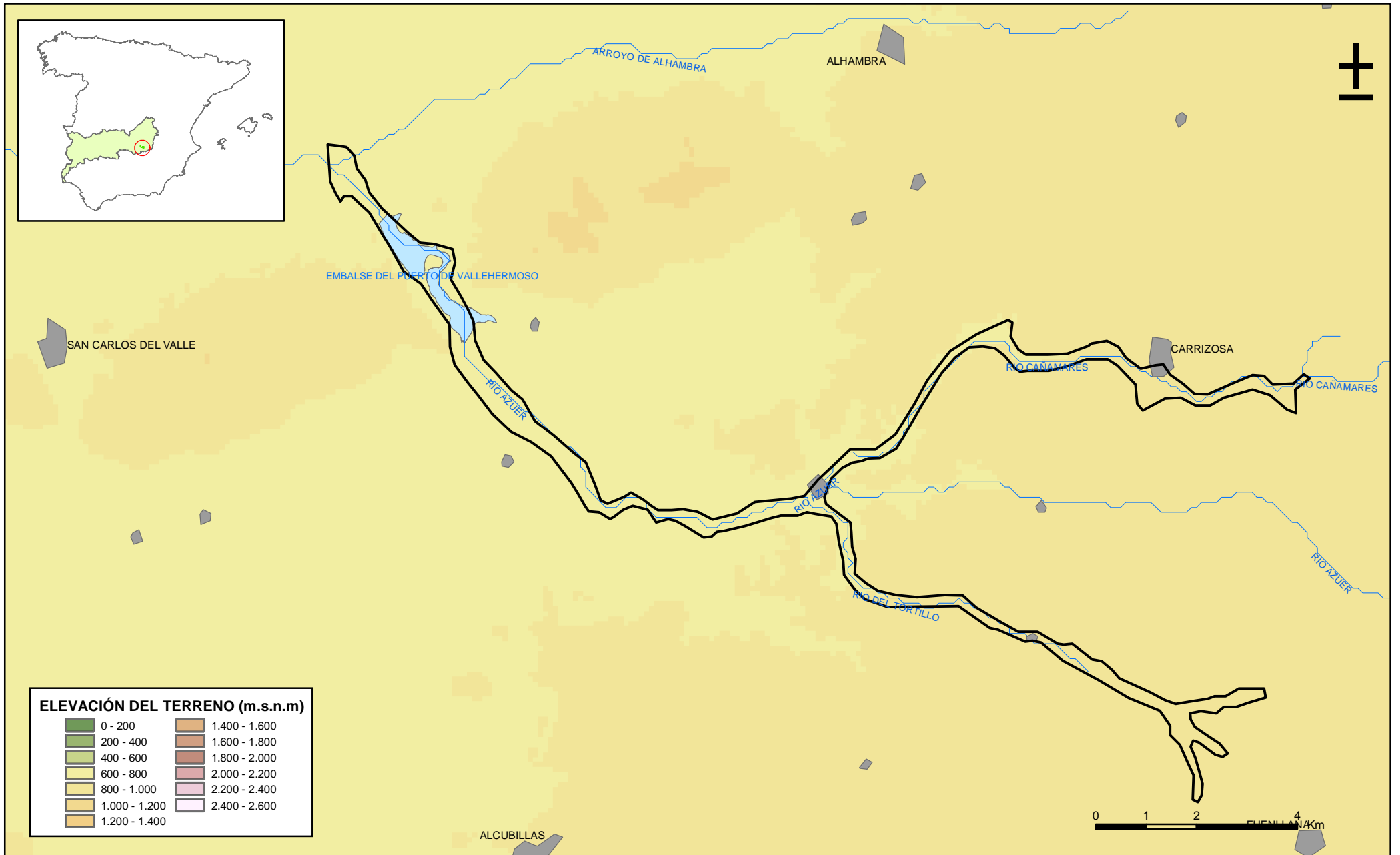
Mapa 1.2. Mapa digital de elevaciones de la masa Aluvial del Azuer (041012)
