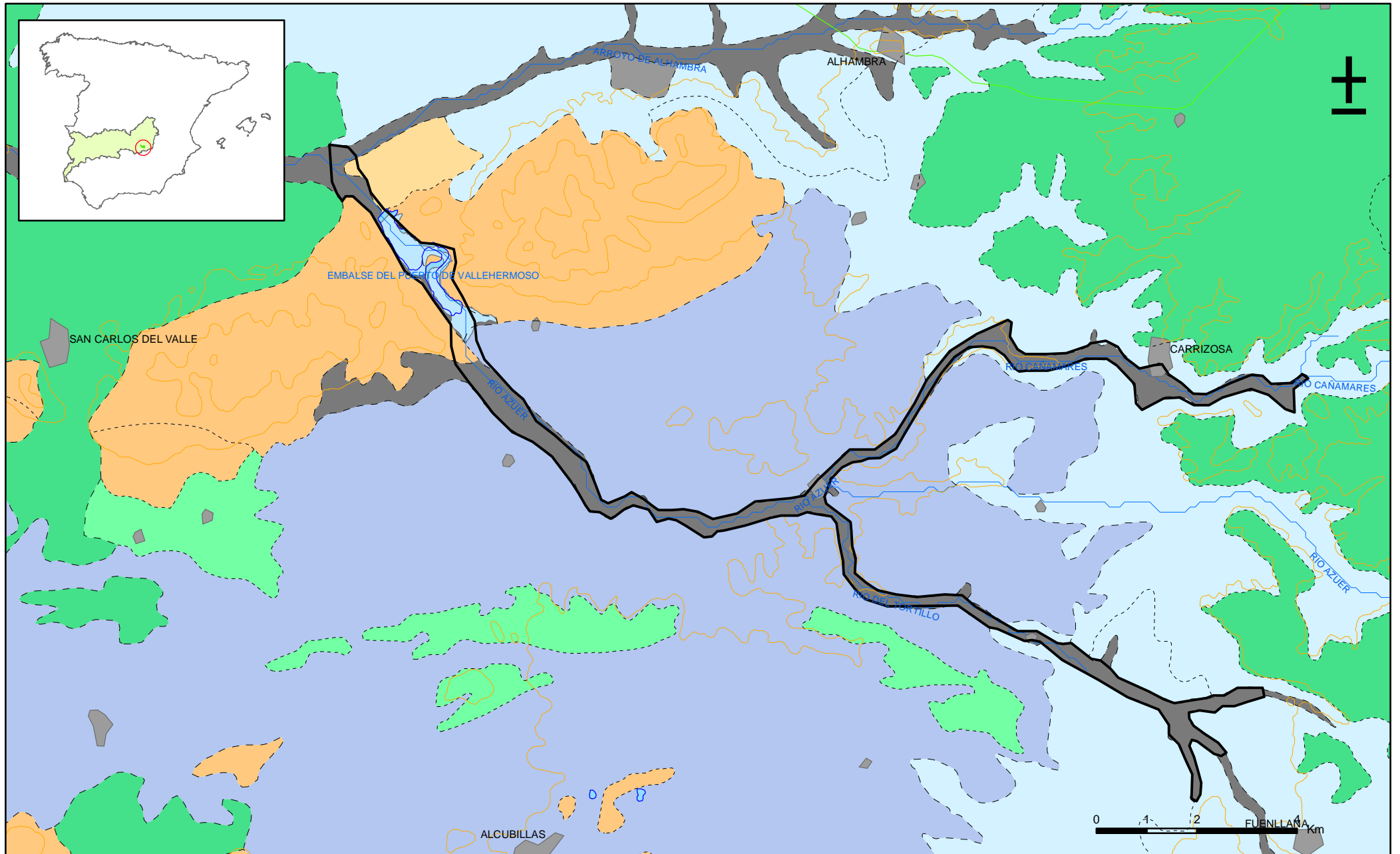
Mapa 3.1. Mapa de permeabilidades según litología de la masa Aluvial del Azuer (041012)
