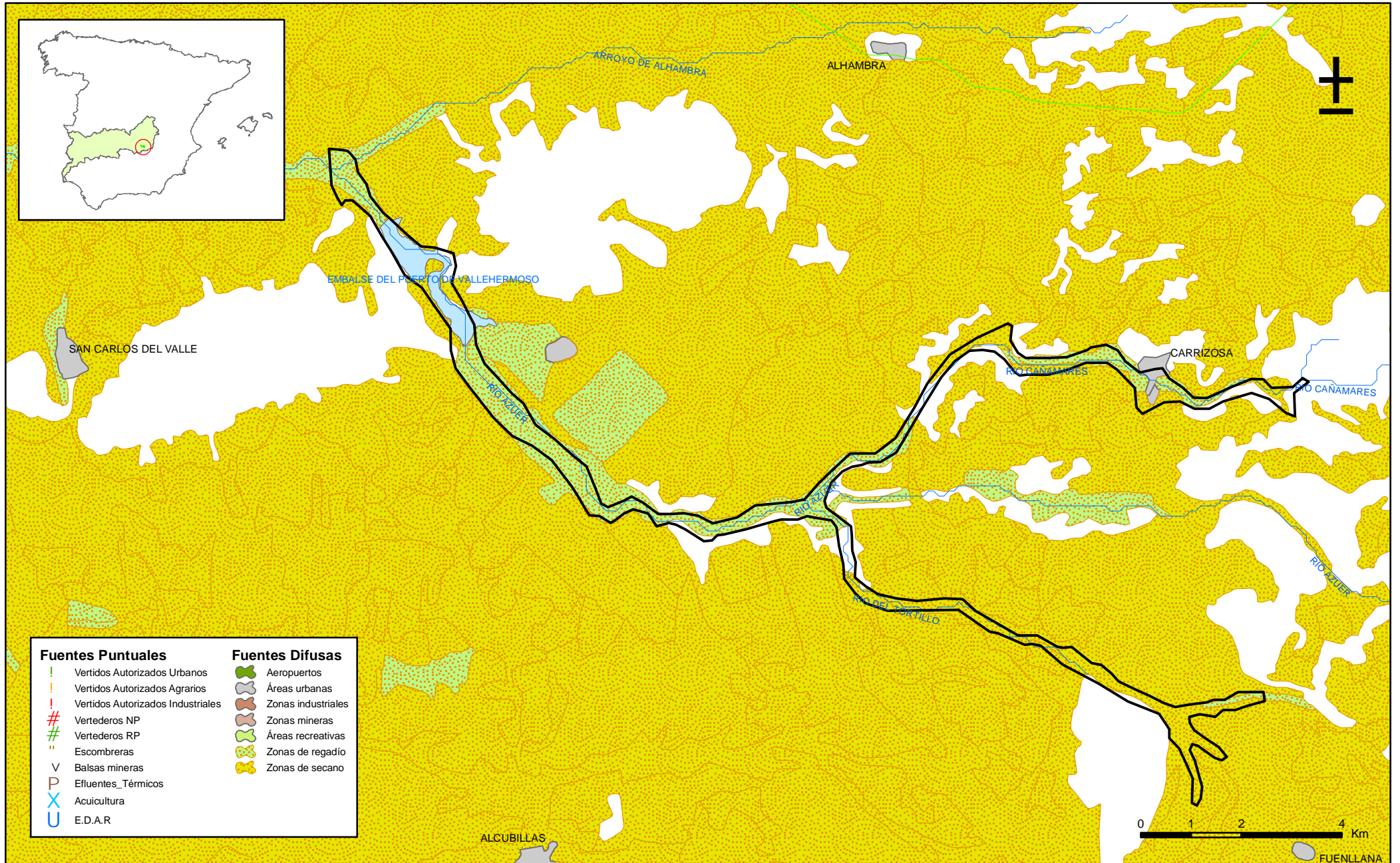
Mapa 14.1. Mapa de actividades potencialmente contaminantes de la masa Aluvial del Azuer (041012)
