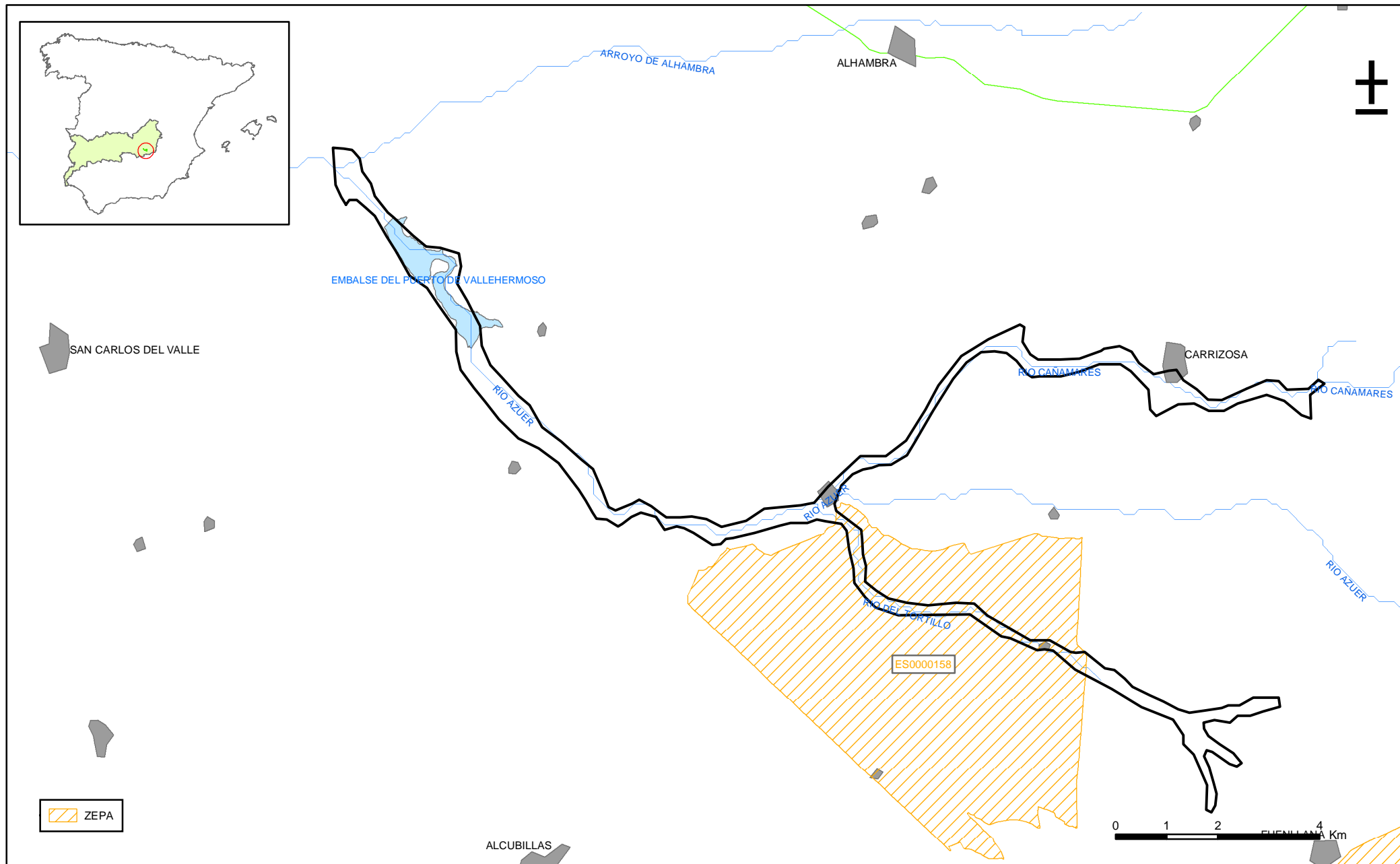
Mapa 6.1. Mapa de situación de ecosistemas dependientes de aguas subterráneas de la masa Aluvial del Azuer (041012)
